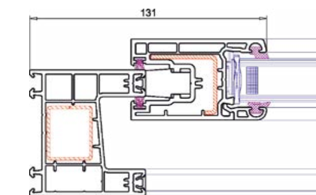
Secção lateral janela
