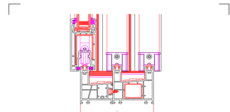
Secção inferior porta
